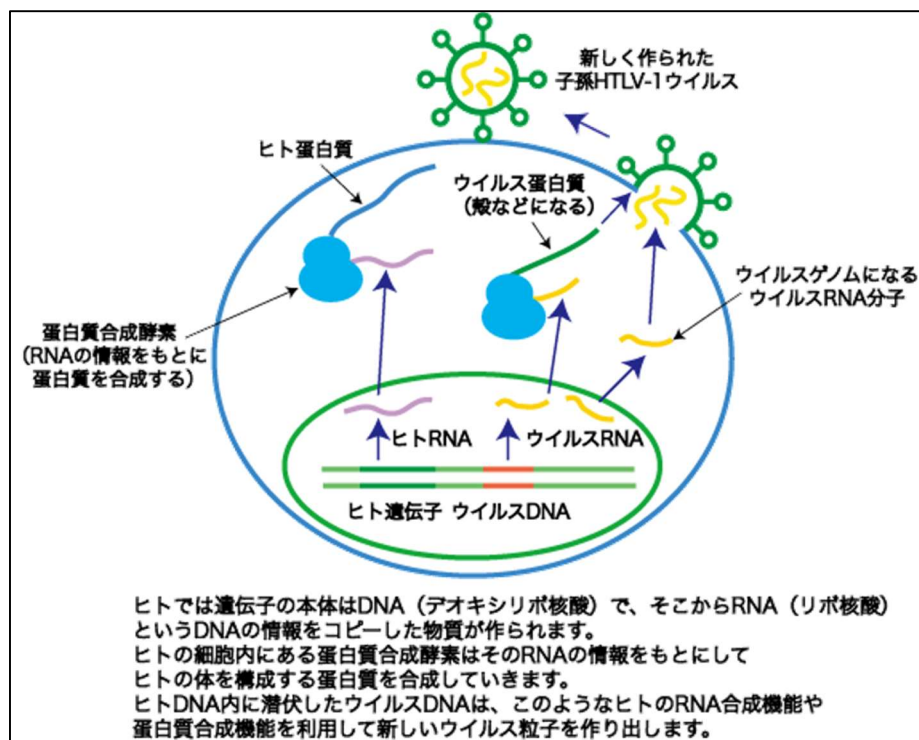
図 2-3. HTLV-1 の増殖（文献 2 より）
